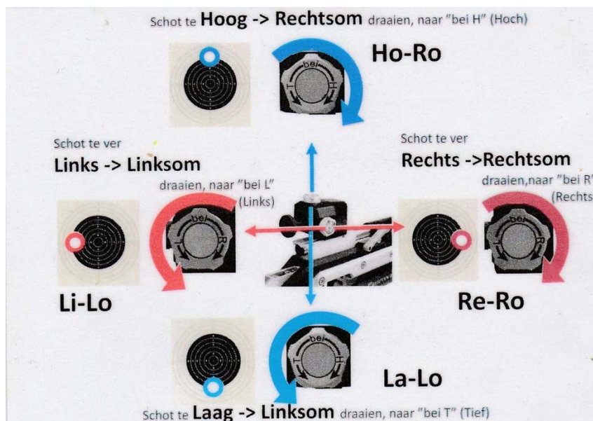
Bijstellen diopter
